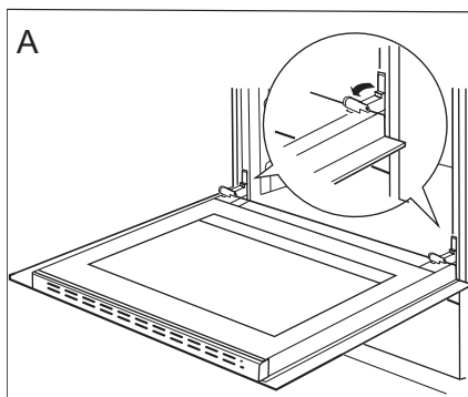
Uppdragning av säkerhetsspärr till gångjärn
